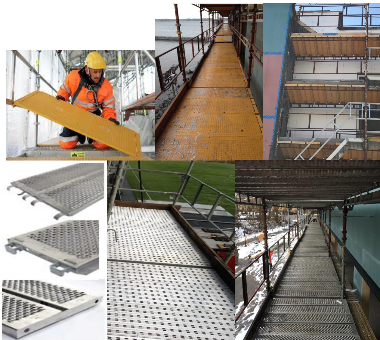
Figur 1 Illustrasjon på ulike godkjente stillaslemmer. Plast og aluminium.
